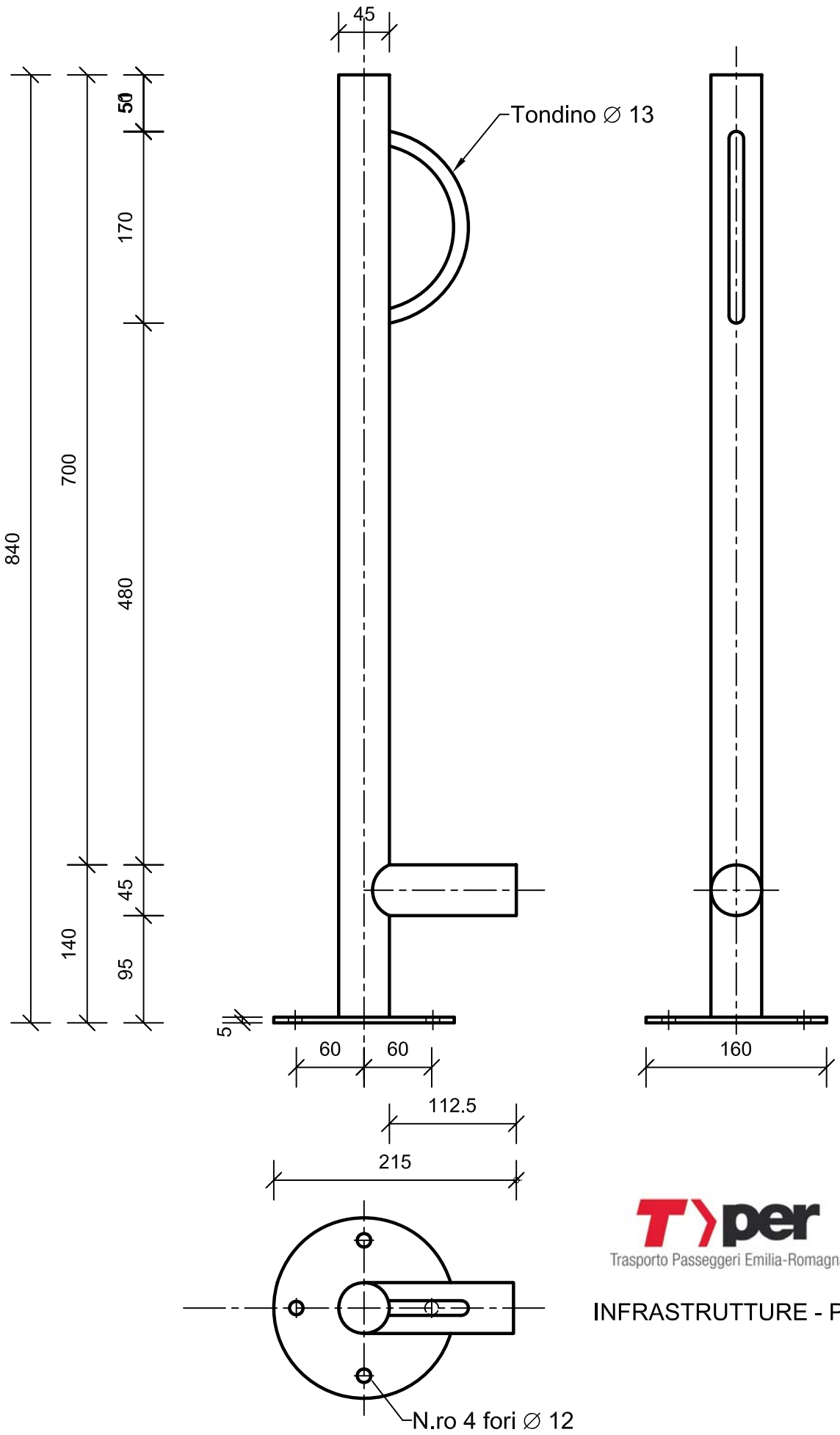
MONTANTE LATERALE scala 1:5
