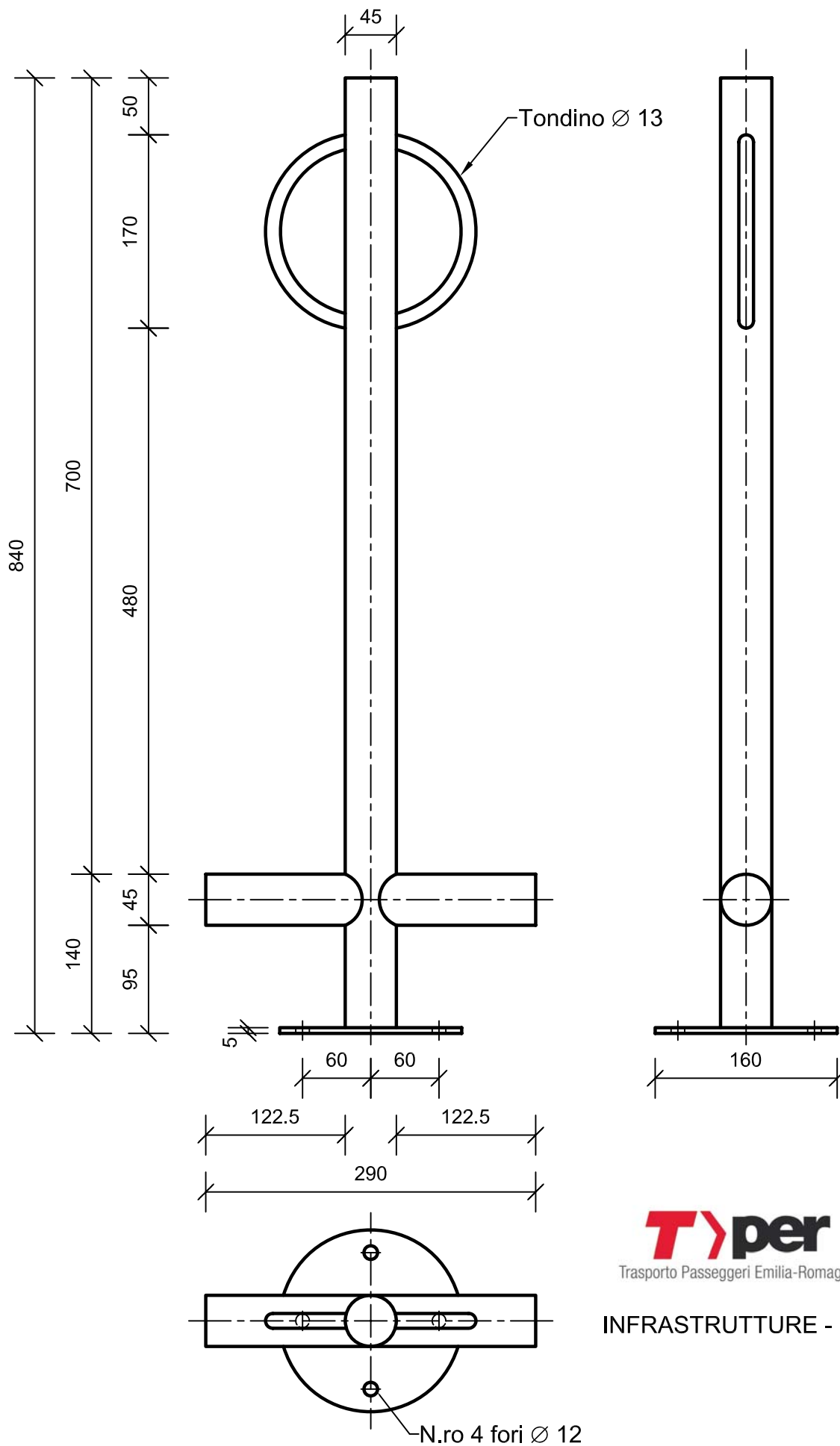
MONTANTE CENTRALE scala 1:5
