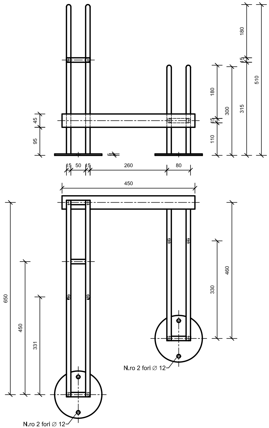
MODULO RASTRELLIERA scala 1:5
